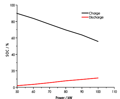
3、不同功率下的充放电截止SOC曲线 Cutoff SOC with different power
