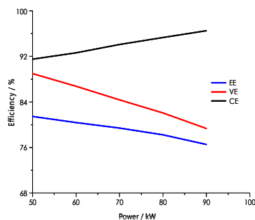
1、不同功率下的充放电特性曲线 Charge/Discharge Performance with different power
